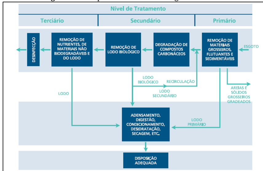
Fluxograma 1 - Etapas do tratamento de esgotos em uma ETE
