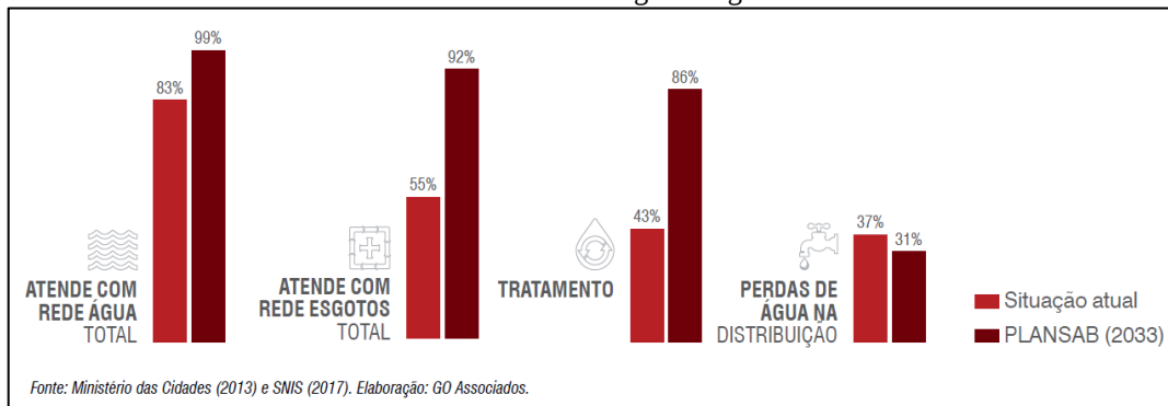
Gráfico 30 - Indicadores de água e esgoto no Brasil
